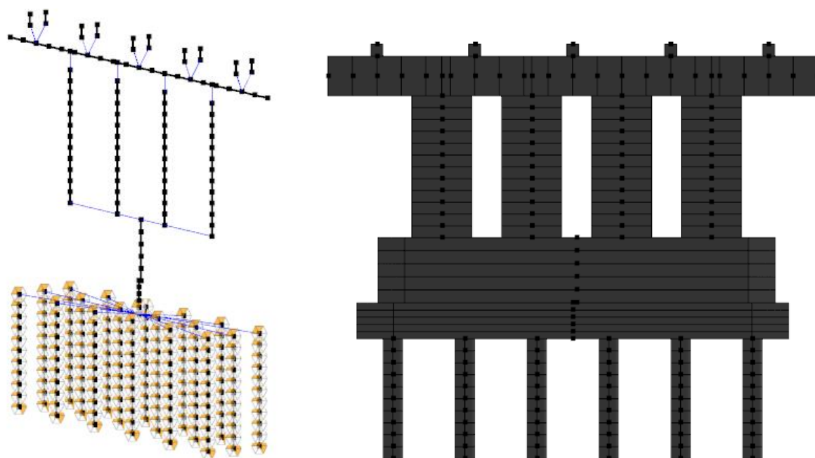
Рисунок 4.3 – Расчетная модель опоры, созданная с помощью мастера создания конструкций
