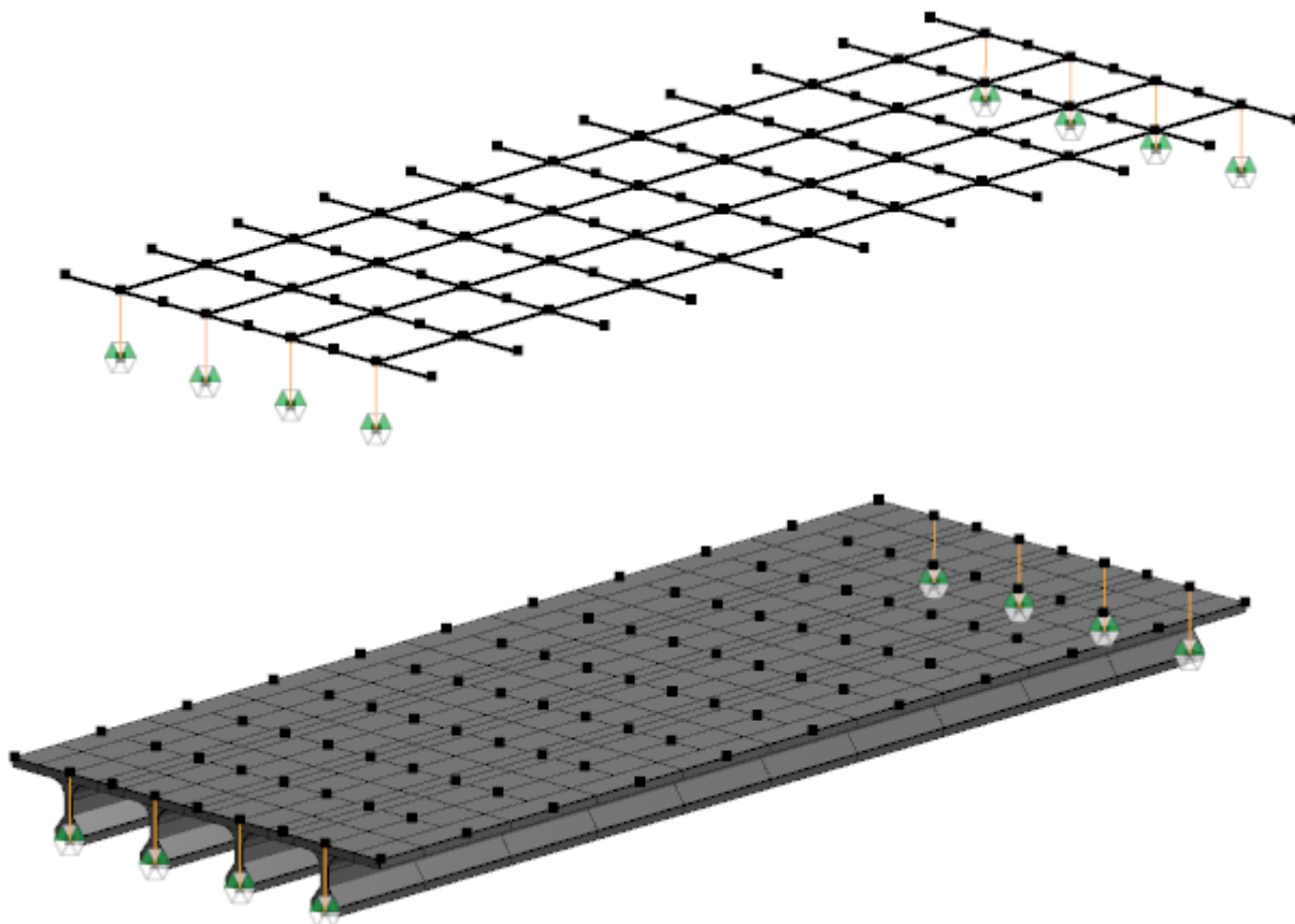
Рисунок 4.5 – Расчетная модель пролетного строения, созданная с помощью мастера создания конструкций
