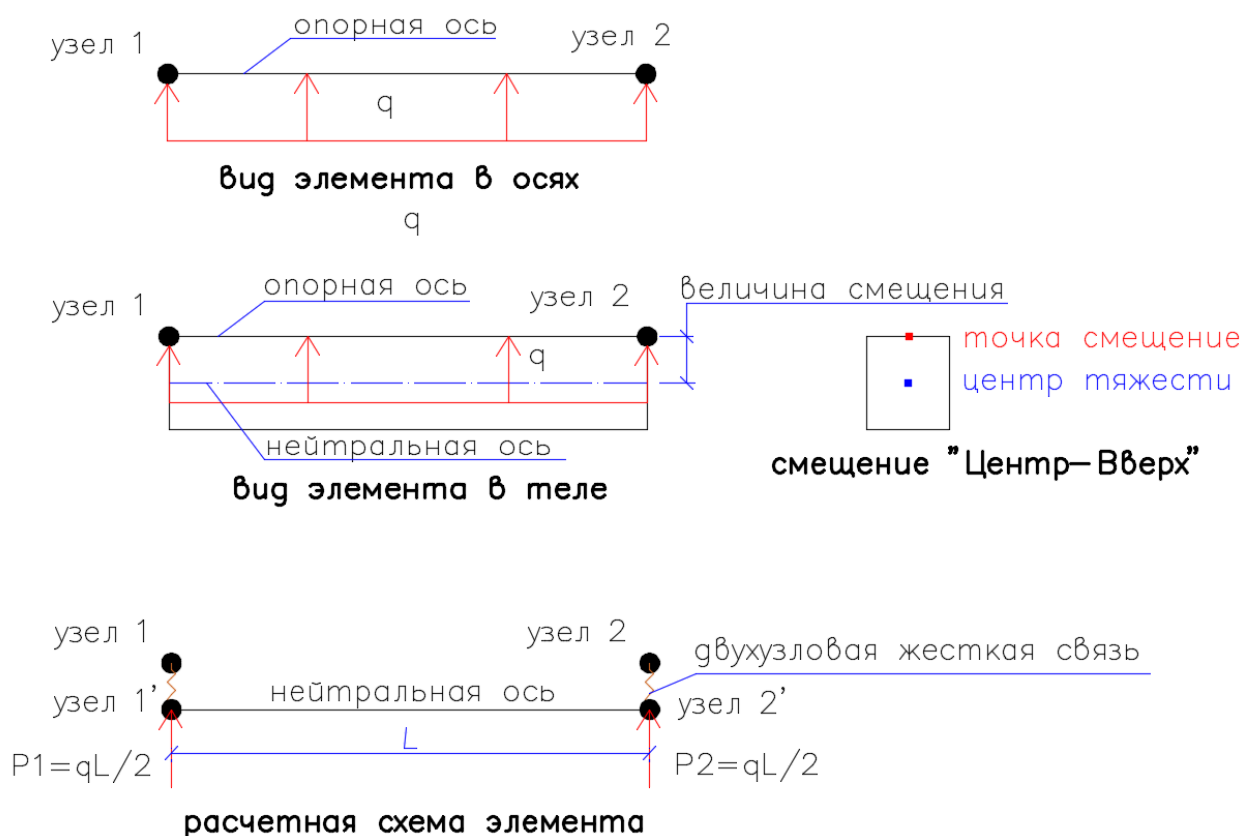
Рисунок 2.40 – Влияние смещения на приложение распределенных сил
