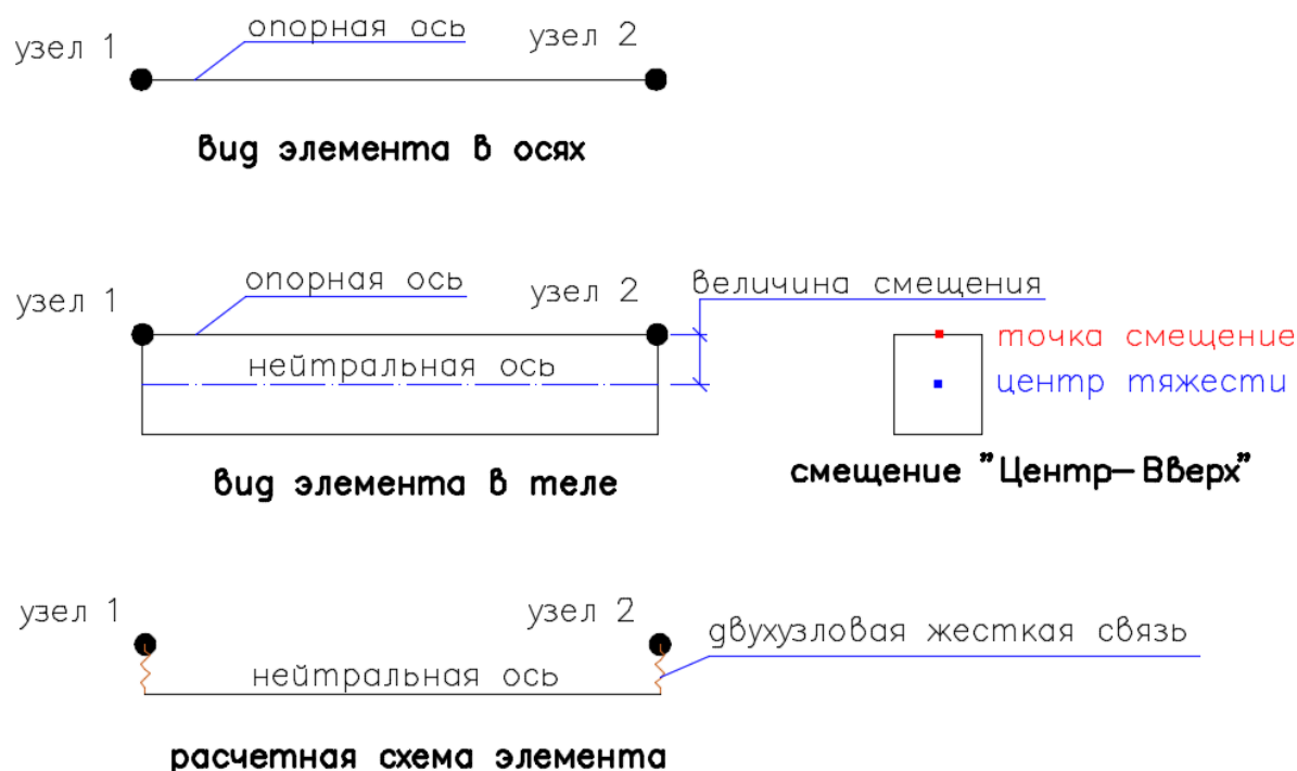
Рисунок 2.38 – Влияние смещения на расчетную схему элемента
